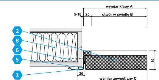
Detal B – Sposób montażu w ścianie lekkiej
