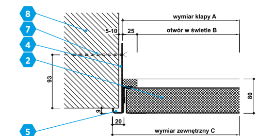
Detal C – Sposób montażu w ścianie masywnej
