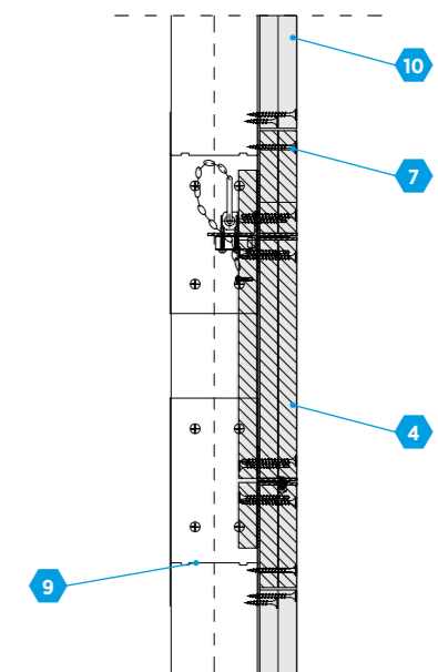
Detal A - Sposób montażu w ścianie g-k (przekrój)
