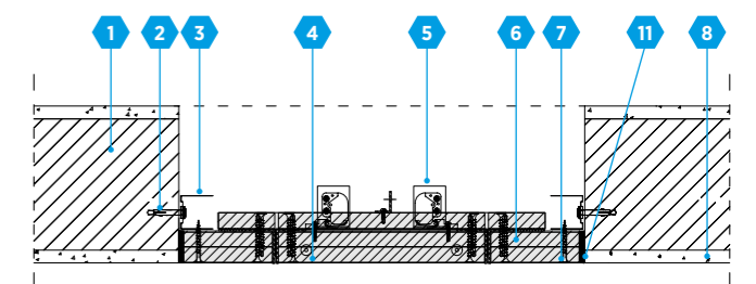
Detal B - Sposób montażu w ścianie masywnej (rzut)
