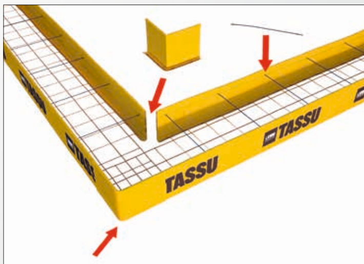
Elementy wycięte na początku prac montażowych ze ścianek formy służą do wykonania elementów narożnych oraz ewentualnych form kolumnowych.
