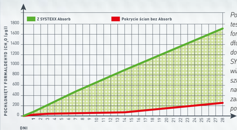
SYSTEXX Active Absorb w porównaniu do tradycyjnych tapet
